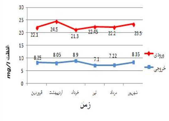
نمودار ۳: روند تغییرات نیترات در مراحل نمونه برداری
