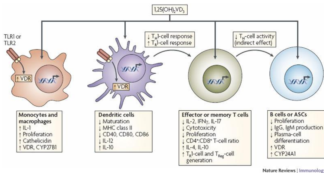
شکل ۲: به طور مختصر نمایی از نقش تنظیمی و تعدیلی 1,25(\text{OH})_2\text{D}_3 را آشکار می‌کند [۳۱].
