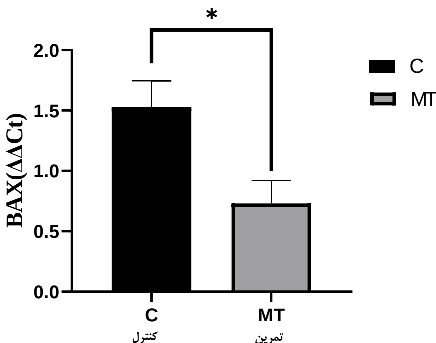
شکل ۱. میزان نسبی بیان ژن BAX در گروه‌های تمرین تداومی (MT) و کنترل (C) * تفاوت معنادار گروه تمرین با کنترل ( P=0/012 ) (میانگین ± انحراف استاندارد)
