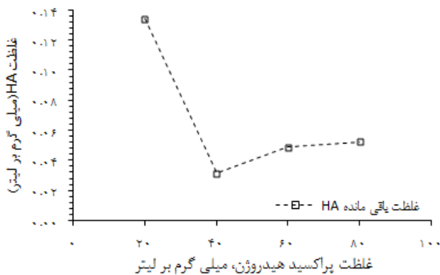
شکل ۲: غلظت هیومیک اسید باقی مانده در زمان استفاده از غلظت های مختلف پراکسید هیدروژن ( زمان اکسیداسیون ۴۰ دقیقه، pH=۳، ۲ mg/l ) ([Fe +2 ]=۴ mg/l، [HA]=)
