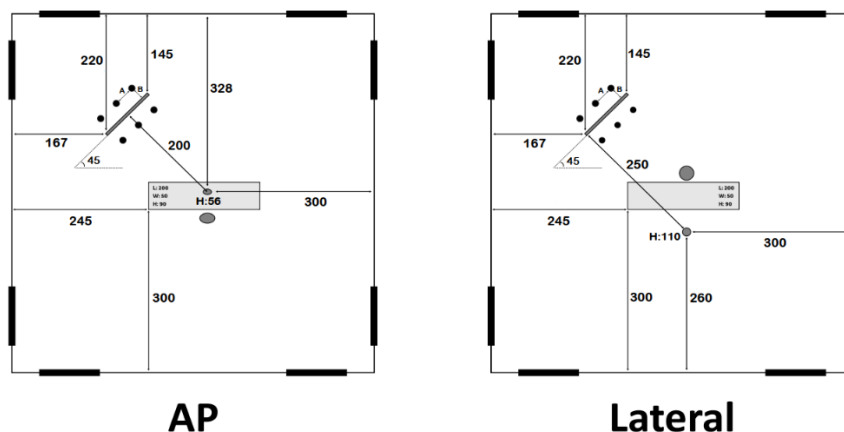
شکل ۱: طرح شماتیکی از اتاق عمل و مختصات قرارگیری دستگاه، دیوار، مولازها و تخت جراحی که تمام اعداد برحسب سانتی متر است. تخت جراحی ۲۰۰ سانتی متر طول، ۵۰ سانتی متر عرض و ۹۰ سانتی متر ارتفاع از سطح زمین دارد. A: فاصله دو مولاز از یکدیگر که برابر است با ۲۸ سانتی متر. B: فاصله مولاز از دیوار سربی که برابر است با ۲۰ سانتی متر. H: فاصله منبع تولید اشعه دستگاه C-arm از سطح زمین.
