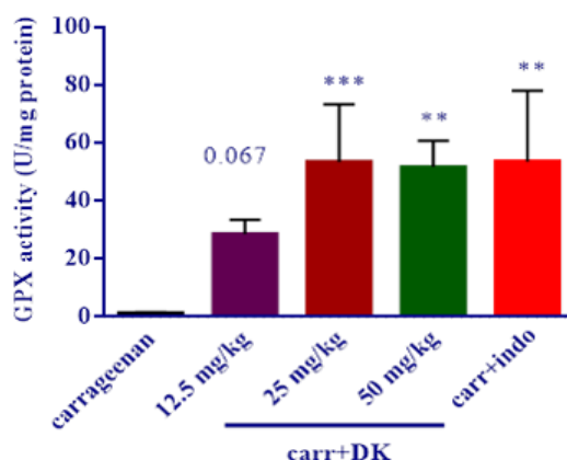
شکل ۶: فعالیت GPX پنجه چهار ساعت پس از تزریق عصاره اتانولی D.kotschy در دوزهای مختلف و *** نشان دهنده تفاوت معناداری در مقایسه با گروه تزریق شده با کاراژنین است ( P < 0.001 ).
