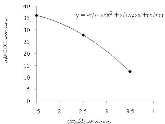
شکل ۲: ارتباط زمان ماند هیدرولیکی و درصد حذف
