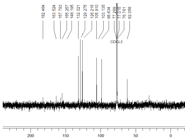
شکل 3: طیف کربن NMR ترکیب 1 (wogonin)
