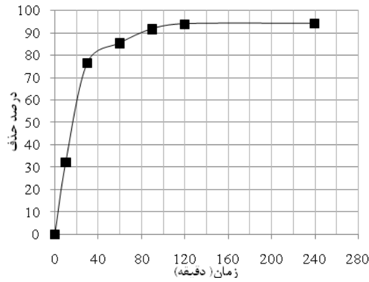
نمودار ۱: تاثیر زمان های مختلف تماس روی میزان راندمان جذب رنگ انتخابی توسط خاکستر
