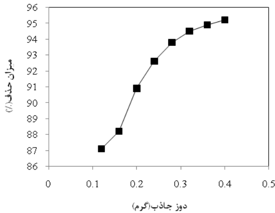
نمودار ۳: تاثیر دوزهای مختلف خاکستر پوست پرتقال روی راندمان جذب رنگ انتخابی ( \text{pH} بهینه 2.9 ، \text{mg/L} و C_0=10 ، t=90 \text{ min} )
