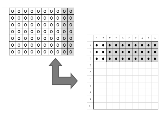
شکل ۵: مفهوم ویژگی تست
