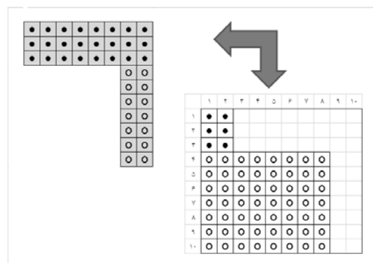
شکل ۸: مفهوم ارزش اخباری مثبت
