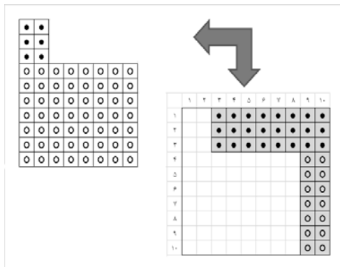
شکل ۹: مفهوم ارزش اخباری منفی
