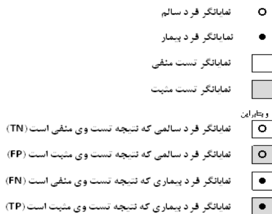
شکل ۱: راهنمای نمادهای مورد استفاده در مقاله
