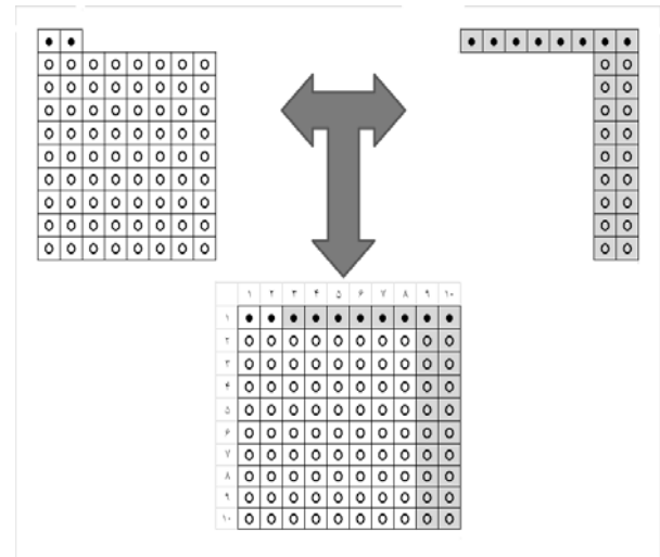
شکل ۱۰: نتیجه تست در جامعه ای با شیوع ۱۰٪
