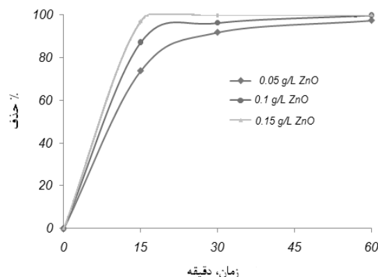
شکل ۱: تأثیر زمان تابش بر روی میزان حذف کروم (VI) (Cr (VI)=۰/۰۵ mg/L, pH=۷)
