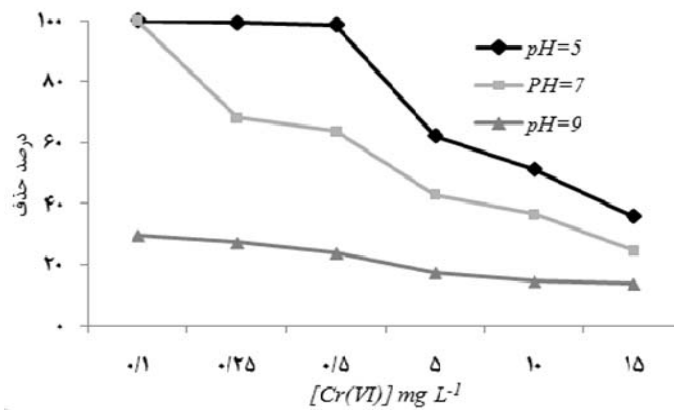
شکل ۴: نمودار غلظت- درصد حذف کروم در pH های مختلف (TiO 2 = ۱۵۰ mg/L، زمان تابش : الف) ۱۵ دقیقه (ب) ۳۰ دقیقه (ج) ۶۰ دقیقه)
