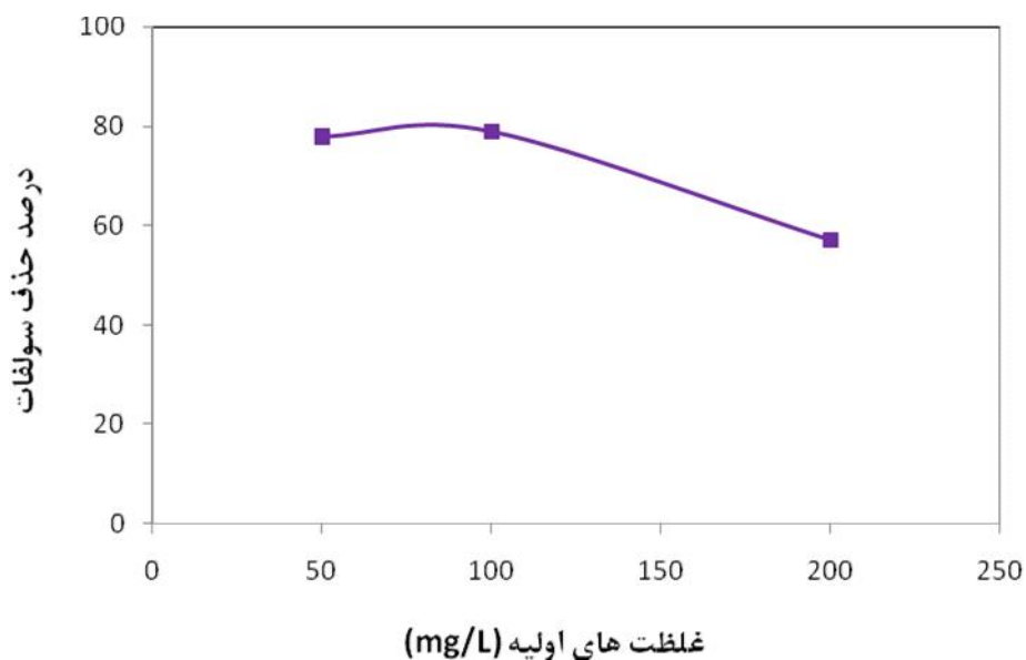
شکل ۳: تأثیر غلظت اولیه سولفات بر میزان حذف از فاز مائی (شرایط: زمان ۱۱۰ دقیقه، جریان اعمالی ۱۶/۶۷ \text{ mA/cm}^2 ، \text{pH } ۷/۲ ).
