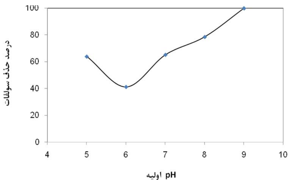
شکل ۴: تأثیر pH اولیه سولفات بر میزان حذف از فاز مائی (شرایط: زمان ۱۱۰ دقیقه، سولفات ۱۰۰ \text{ mg/l} ، جریان اعمالی ۱۶/۶۷ \text{ mA/cm}^2 ).
