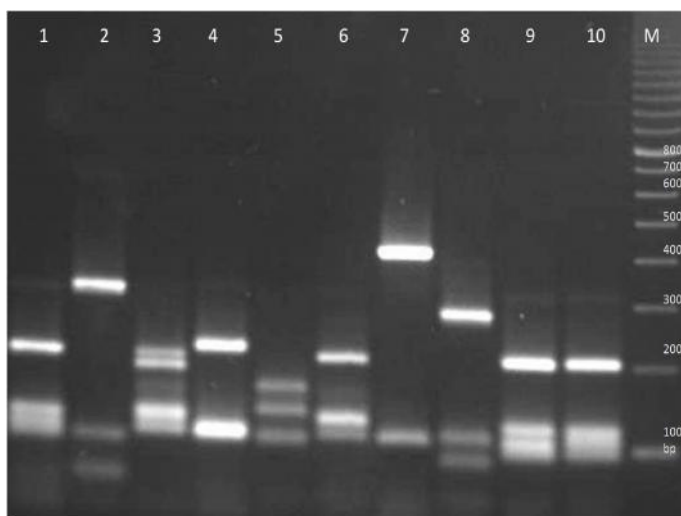
شکل ۲: تصویر الکتروفورز از محصولات PCR-RFLP گونه های استاندارد آسپرژیلوسی که به عنوان الگوی تشخیصی گونه های بالینی آسپرژیلوس در این مطالعه مورد استفاده قرار گرفت. ستون های ۱-۹: آسپرژیلوس فومیگاتوس، آسپرژیلوس فلاووس، آسپرژیلوس نایجر، آسپرژیلوس ترئوس، آسپرژیلوس نیدولانس، آسپرژیلوس کلاواتوس، آسپرژیلوس اوکراسئوس، آسپرژیلوس آمستلئیدامی و آسپرژیلوس فیشری، ستون ۱۰: نتوسارتوریا کوادریسینکتا که الگویی مشابه آسپرژیلوس فومیگاتوس دارد. ستون M مربوط به مارکر نردبانی 100bp می باشد.
