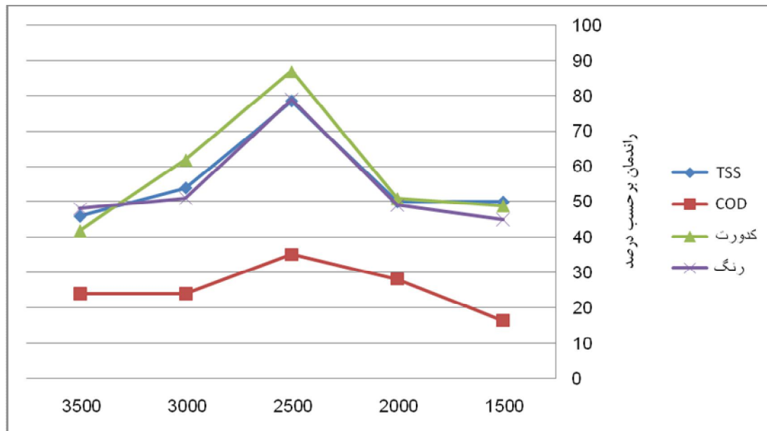
شکل ۵: تاثیر تغییر غلظت در راندمان حذف آلاینده‌ها در pH=۸/۵
