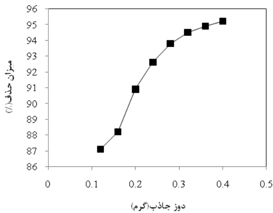
نمودار ۳: تاثیر دوزهای مختلف خاکستر پوست پرتقال روی راندمان جذب رنگ انتخابی ( \text{pH} بهینه 2.9 ، C_0=10 ، t=90 \text{ min} )
