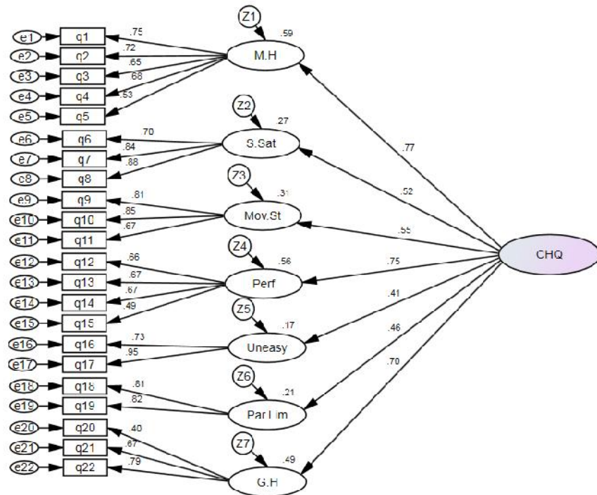
شکل ۲: تحلیل عاملی مرتبه دوم پرسشنامه سلامت کودک (شاخص‌های برازش حاصل از اجرای مدل طبق شکل ۲: GFI=0/869 , CFI=0/907 , RMSEA=0/06 ) تمامی بارهای عاملی مرتبه دوم در سطح کمتر از ۰/۰۰۱ معنادار بودند
