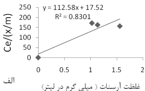
نمودار ۲: ایزوترم لانگموئیر (الف) و فروندلیخ (ب)
