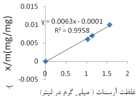
نمودار ۲: ایزوترم لانگموئیر (الف) و فروندلیخ (ب)
