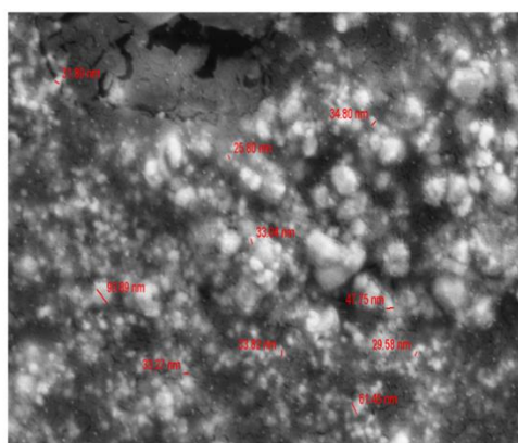
شکل ۱. (الف) تصویر SEM نانوذرات نقره؛ (ب) تصویر آنالیز EDX نانوذرات نقره
