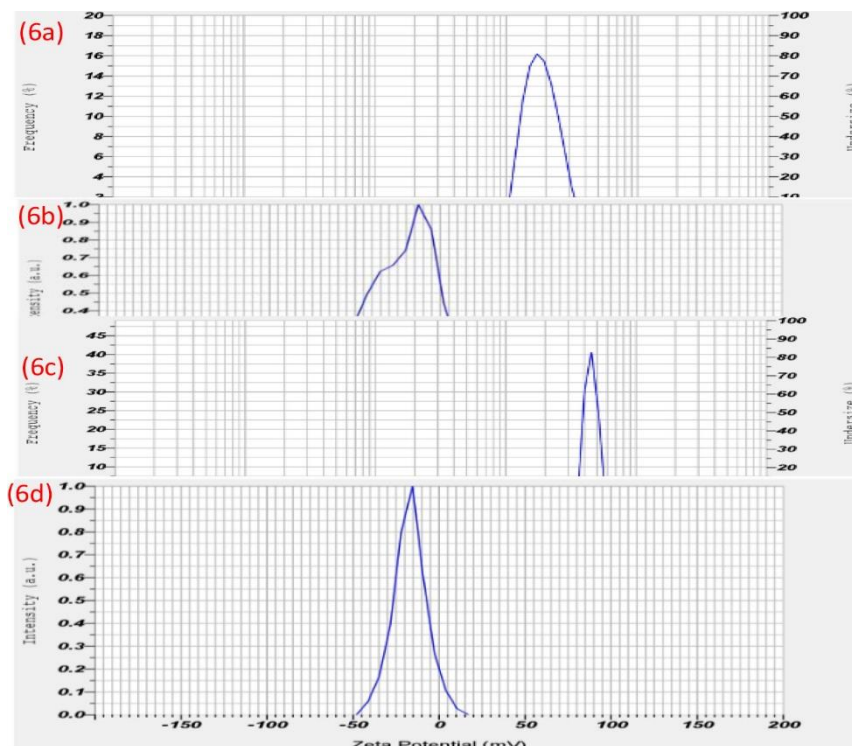
شکل ۶. توزیع اندازه ذرات \text{Co}_3\text{O}_4/\text{Nd}_2\text{O}_3 با استفاده از تکنیک DLS (۶a)، پتانسیل زتا مربوط به نانوذرات \text{Co}_3\text{O}_4/\text{Nd}_2\text{O}_3 و پتانسیل زتا: ۱۹/۶- میلی‌ولت و میانگین تحرک الکتروفوریتیک: ۰/۰۰۱۵۲ سانتی‌متر مربع /Vs)، توزیع اندازه ذرات \text{G-Co}_3\text{O}_4/\text{Nd}_2\text{O}_3 با استفاده از تکنیک DLS (۶c) و میانگین اندازه ذره: ۴۲۵/۵ نانومتر، انحراف معیار اندازه ذره: ۴۴/۰ نانومتر و مقدار مد داده‌ها: ۴۲۳/۷ نانومتر) و پتانسیل زتا مربوط به نانوذرات \text{G-Co}_3\text{O}_4/\text{Nd}_2\text{O}_3 (۶d)، پتانسیل زتا: ۱۷/۰- میلی‌ولت، میانگین تحرک الکتروفوریتیک: ۰/۰۰۱۳۲ \text{cm}^2/\text{Vs} )
