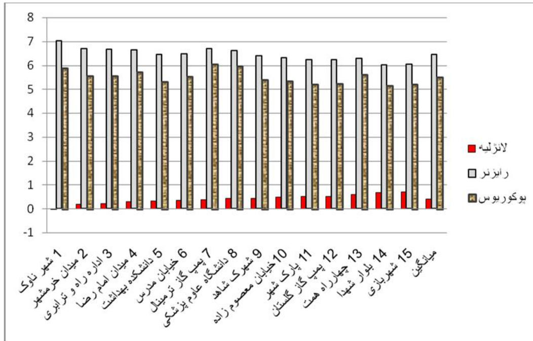
نمودار ۱: شاخص‌های لانتانیم، رایزنر و پوکوریوس آب در شبکه آبرسانی شهر بجنورد در طول دوره بررسی
