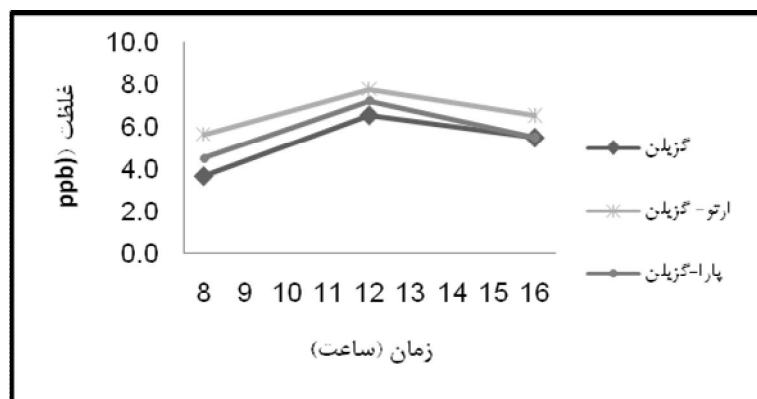
شکل ۲: تغییرات روزانه غلظت گزیلین، ارتو-گزیلین و پارا-گزیلین در سال ۱۳۹۰
