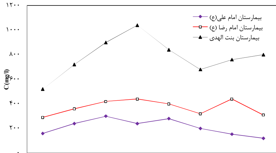
شکل ۲: روند تغییرات شاخص COD در بیمارستان‌های مورد مطالعه نیمه اول تیر ۹۲ نیمه دوم خرداد ۹۲ نیمه اول خرداد ۹۲ نیمه دوم اردیبهشت ۹۲ نیمه اول اردیبهشت ۹۲ نیمه دوم فروردین ۹۲ نیمه اول فروردین ۹۲ نیمه دوم اسفند ۹۱ زمان
